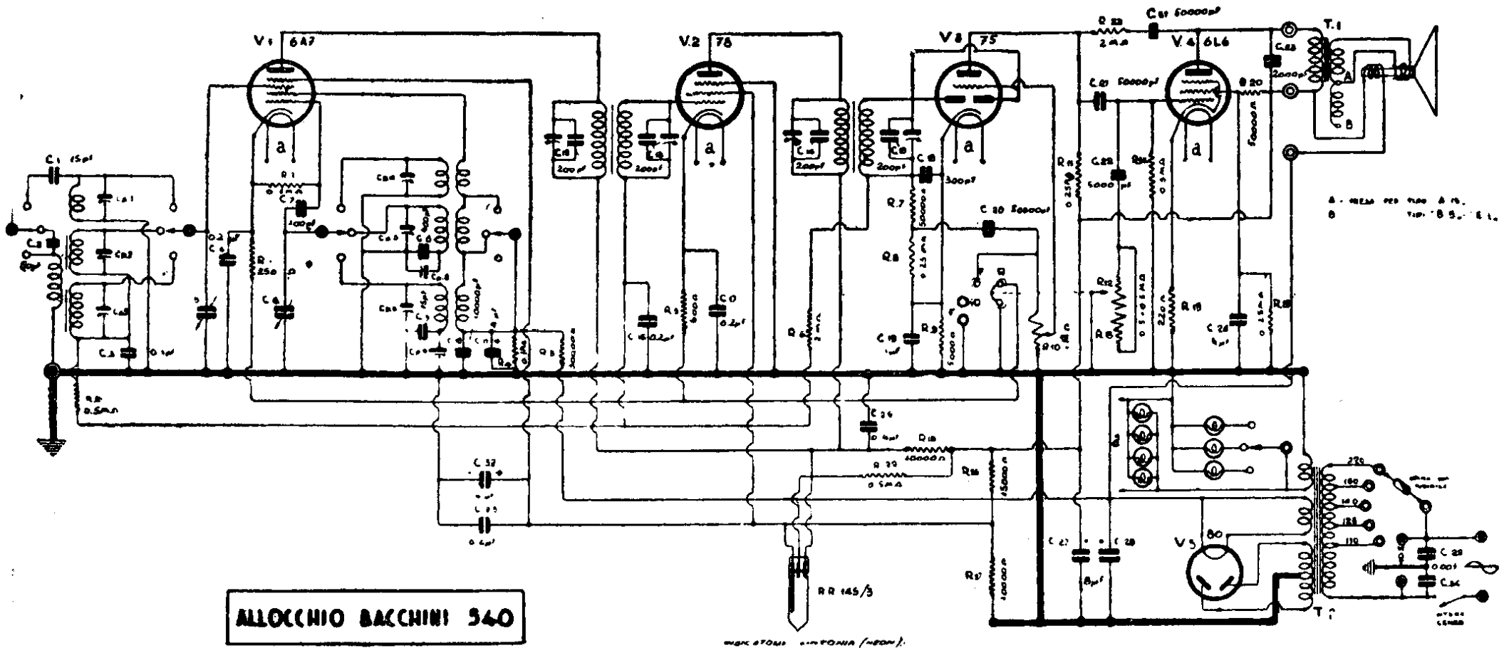
ALLOCCHIO, BACCHINI e Co - Mod 540 R e 540 G - Produzione 1938-39 - Media frequenza 425 kHz.
